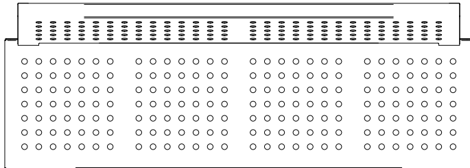
Yan Görünüş / Side View
